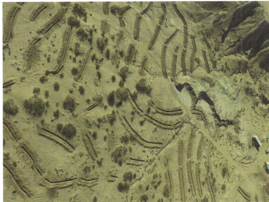
Imagen 12. Vista aérea de las zanjas trinchera
