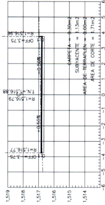
ESTACION 3+003.70 ESCALA HORIZONTAL 1 : 100 ESCALA VERTICAL 1 : 100
