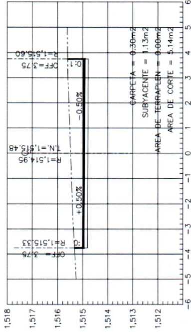
ESTACION 3+028.72 ESCALA HORIZONTAL 1 : 100 ESCALA VERTICAL 1 : 100
