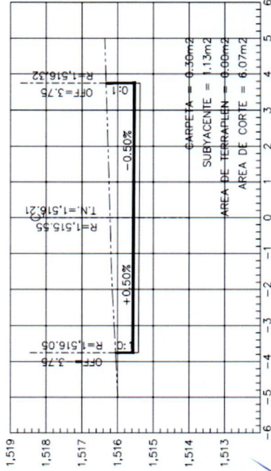
ESTACION 3+020.00 ESCALA HORIZONTAL 1 : 100 ESCALA VERTICAL 1 : 100
